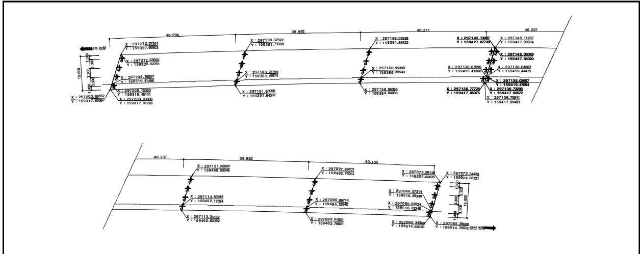
【그림 11.3.1】 교량받침 배치도
