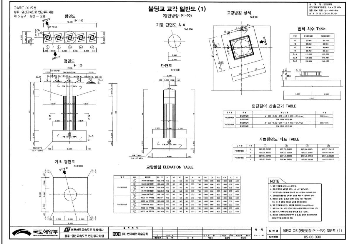
【그림 11.1.7】 교각 일반도
