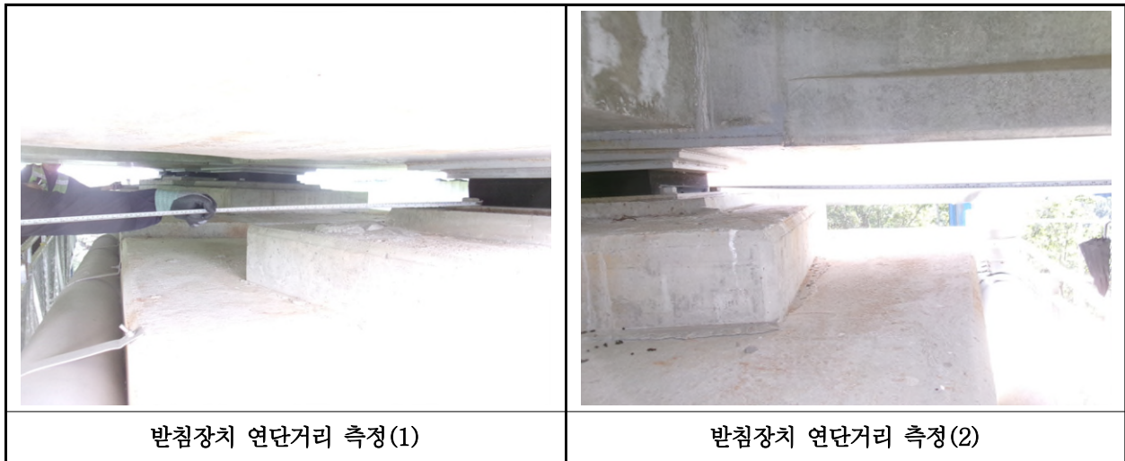
【사진 11.3.39】 교량받침장치 연단거리측정
