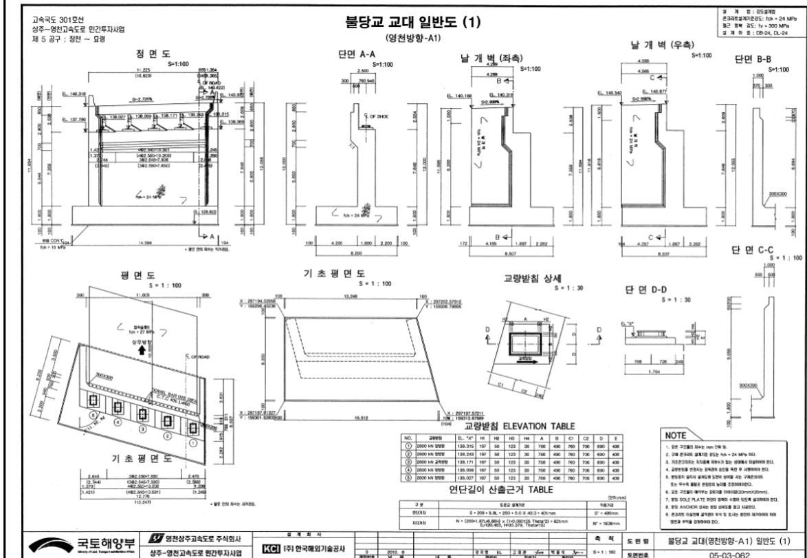
【그림 11.1.6】 교대 일반도
