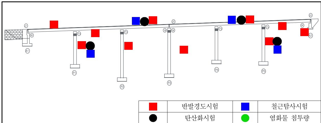
【그림 11.4.2】 콘크리트 내구성조사 위치도(영천방향)
