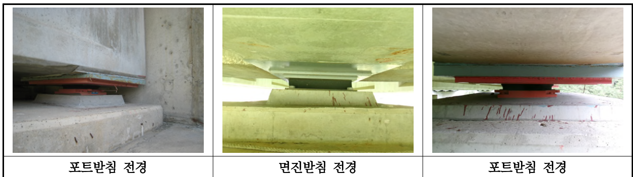
【사진 11.3.12】 교량받침 전경
