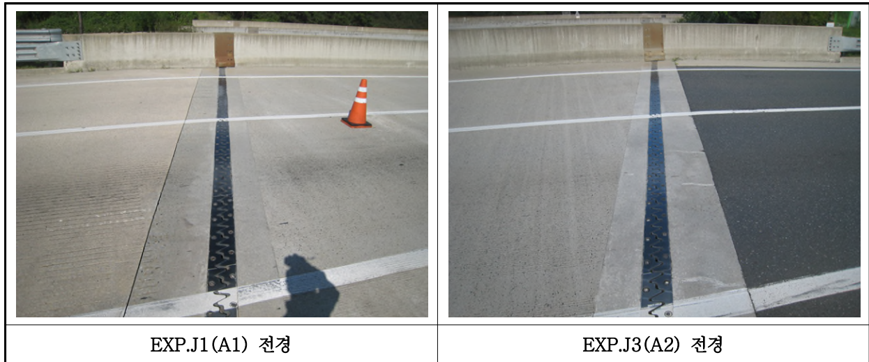
【사진 11.3.41】 신축이음장치 전경
