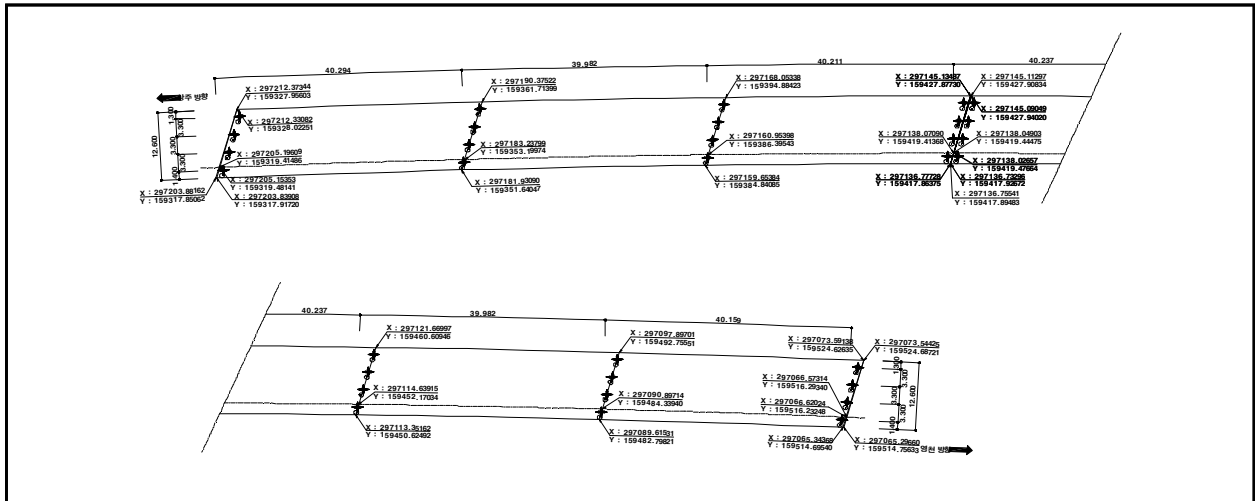
【그림 11.3.3】 교량반침 배치도
