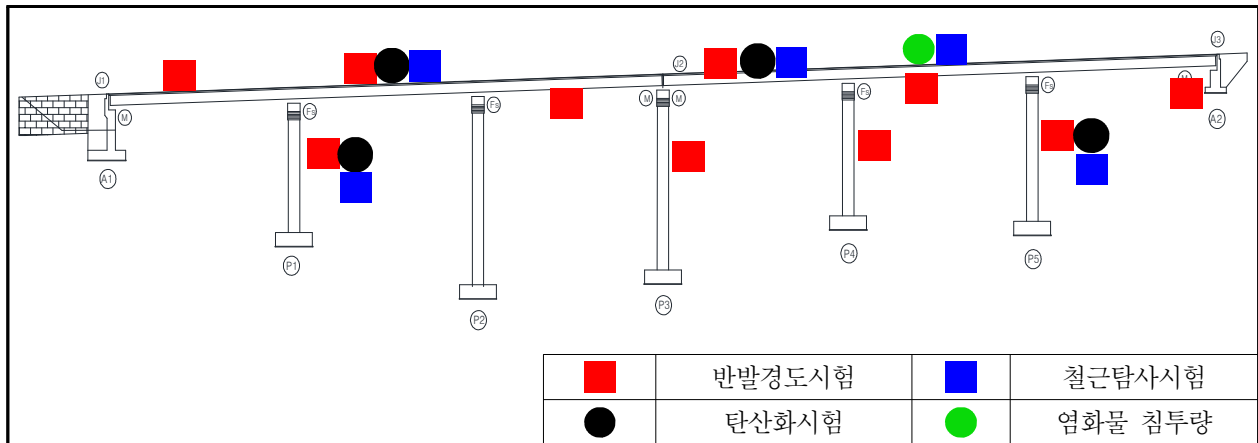
【그림 11.4.1】 콘크리트 내구성조사 위치도(상주방향)
